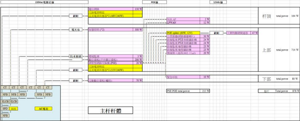
圖 C4-1 Type 3供電網路圖
