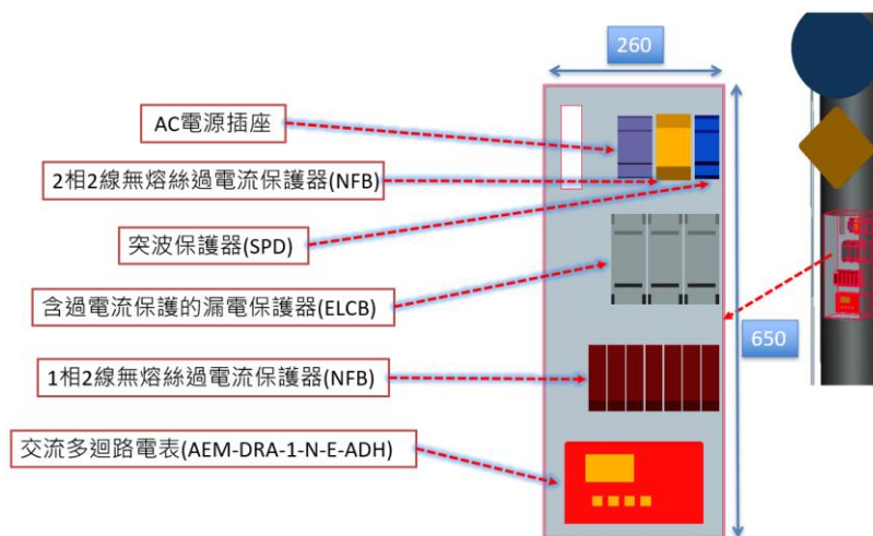
圖5.4.2-2 Type 3分電盤配置圖
