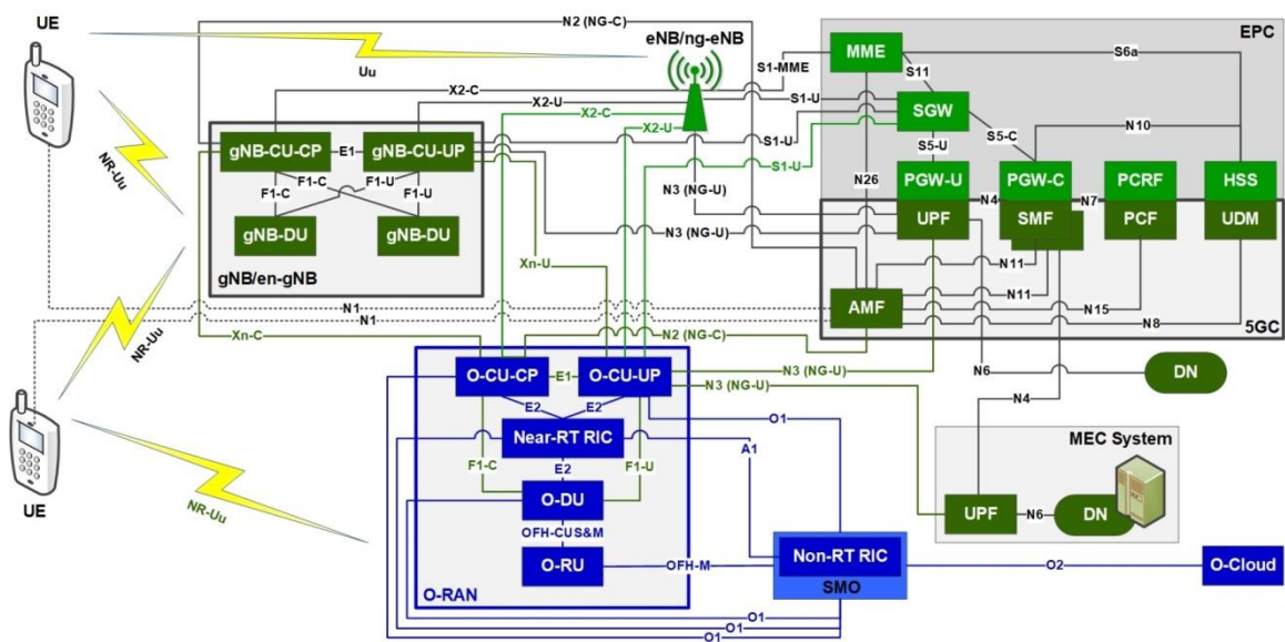
圖6.1.3-1 基站軟體介面標準（引用自O-RAN Alliance）[76]
