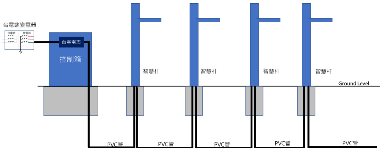
圖4.6.2.3-3 電源管線規劃示意圖
