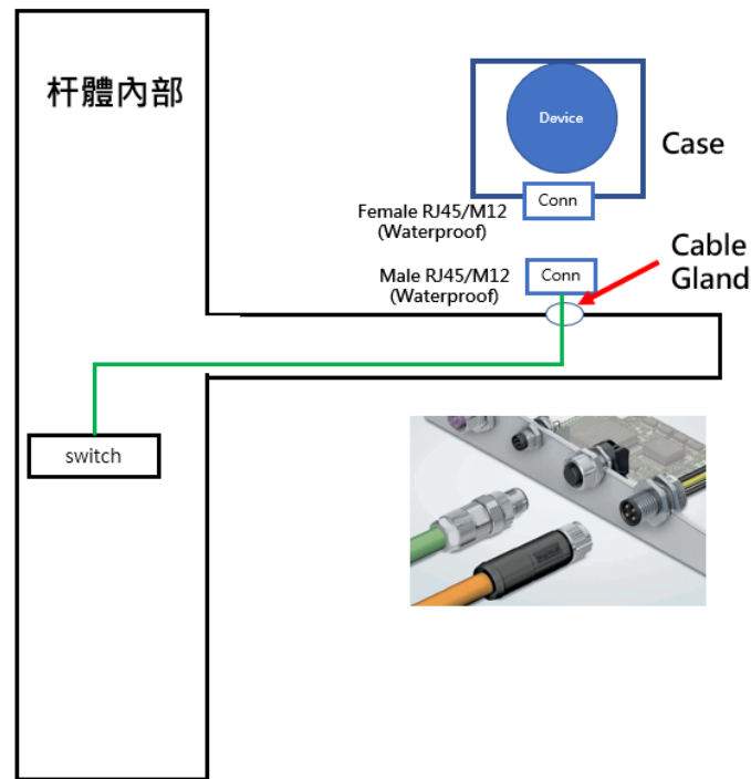
圖 4.3.1.2-5 特定介面在智慧杆上應用示意圖
