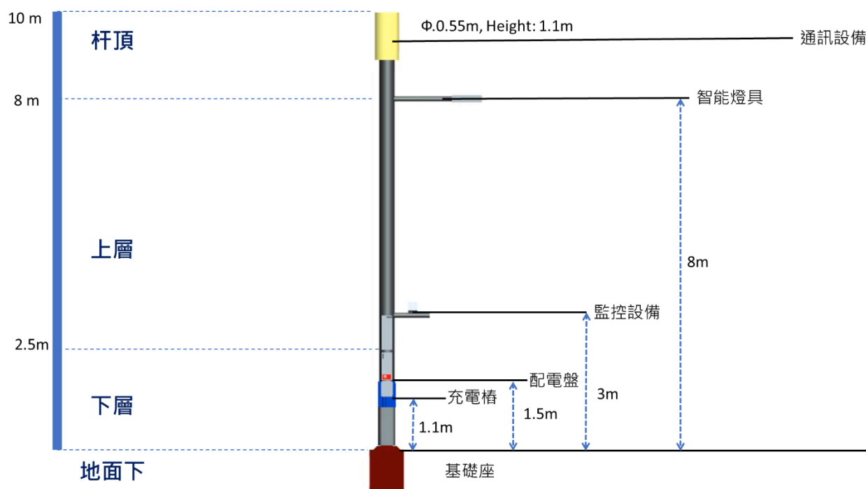
圖 4.2.2.3-1 Type 4 智慧杆掛載設備示意圖
