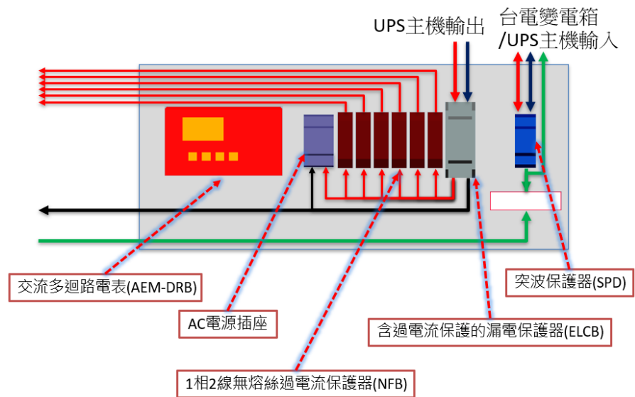
圖 5.1.5-1 控制箱分電盤保護元件及走線參考圖示
