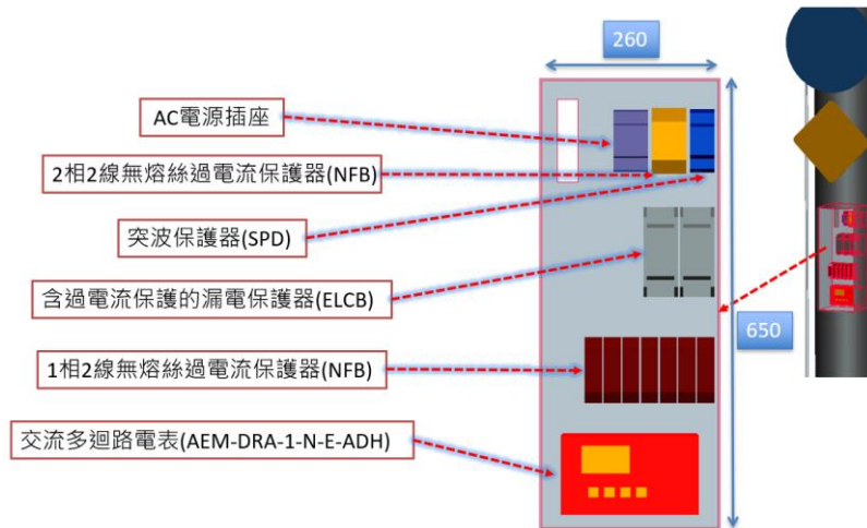
圖5.4.1-2 Type 2分電盤配置圖
