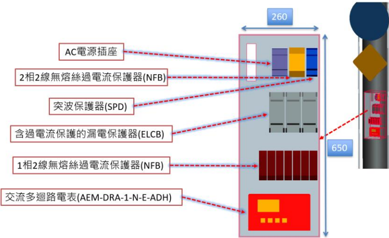
圖 C4-2 Type 3分電盤配置圖
