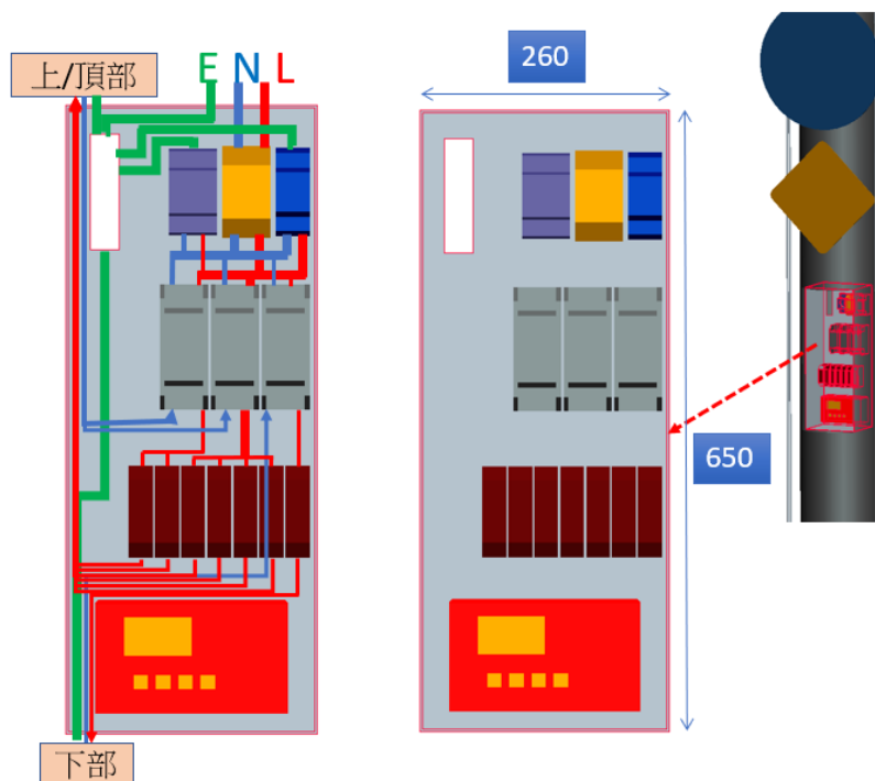
圖5.1.4-1 分電盤配置及走線規畫
