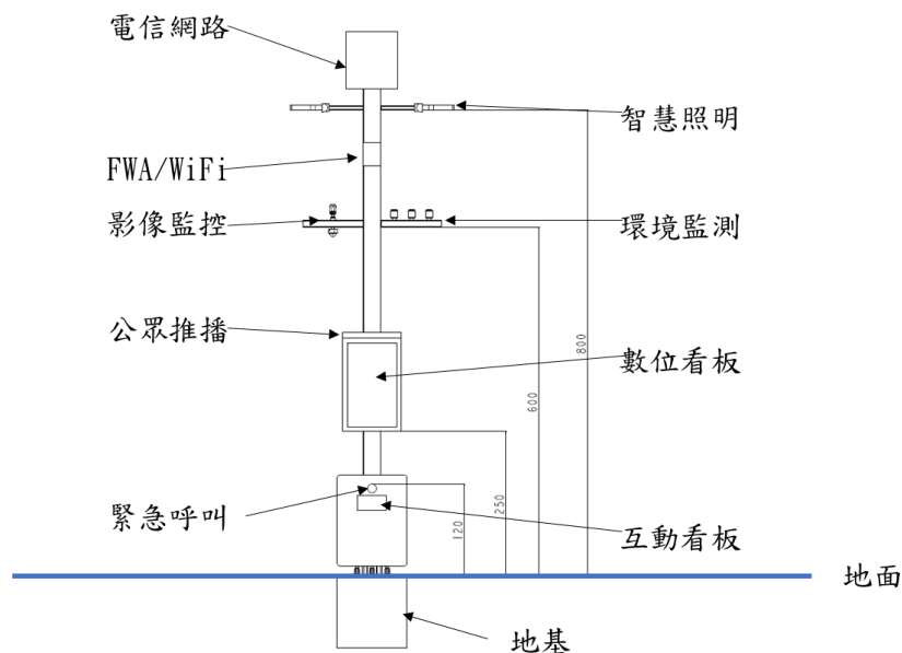
圖 4.2.2.2-1 Type 3 智慧電杆示意圖
