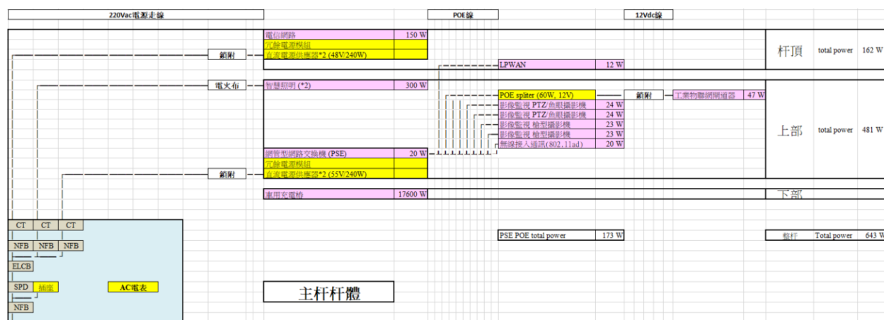
圖5.4.3-1 Type 4供電網路圖
