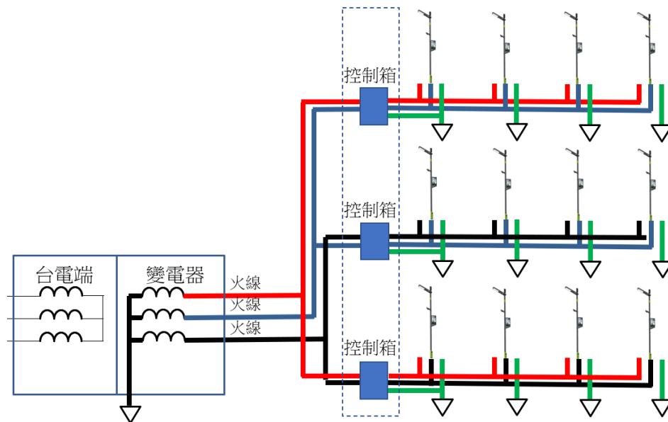
圖 5.1.1-1 智慧杆電力輸入迴路
