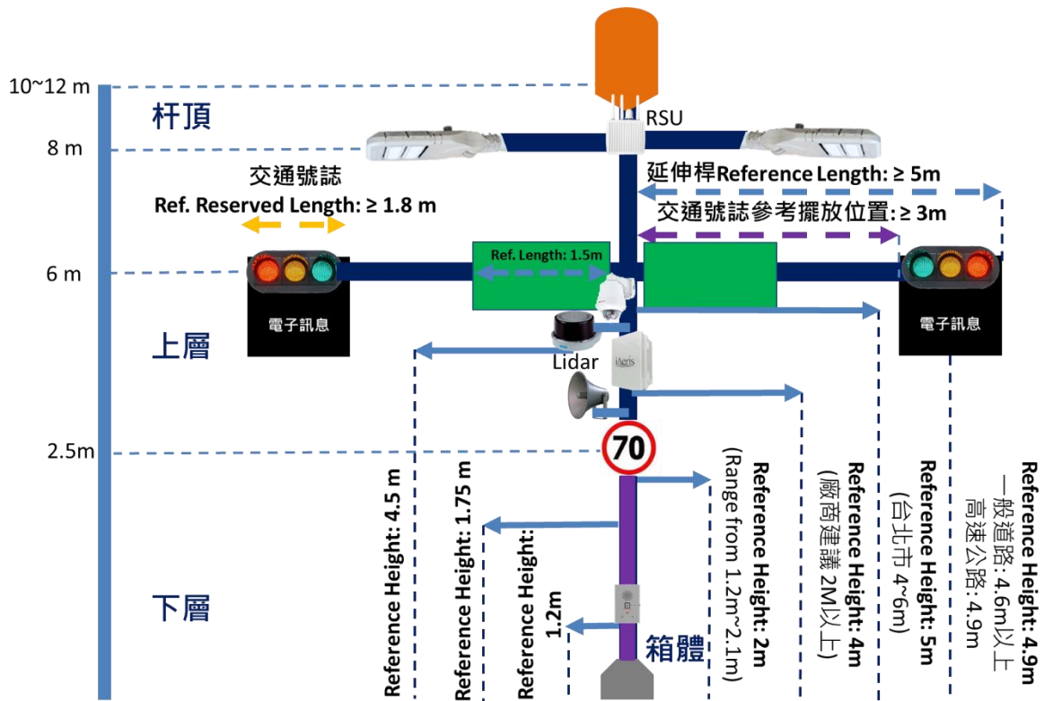
圖 4.2.1-1 5G 智慧杆掛載設備示意圖
