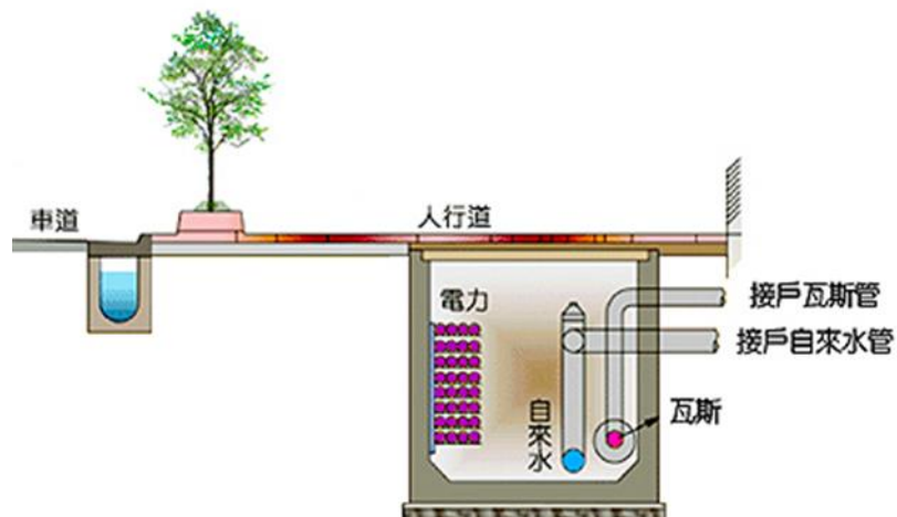
圖 4.6.2.2-2 支管示意圖 [62]
