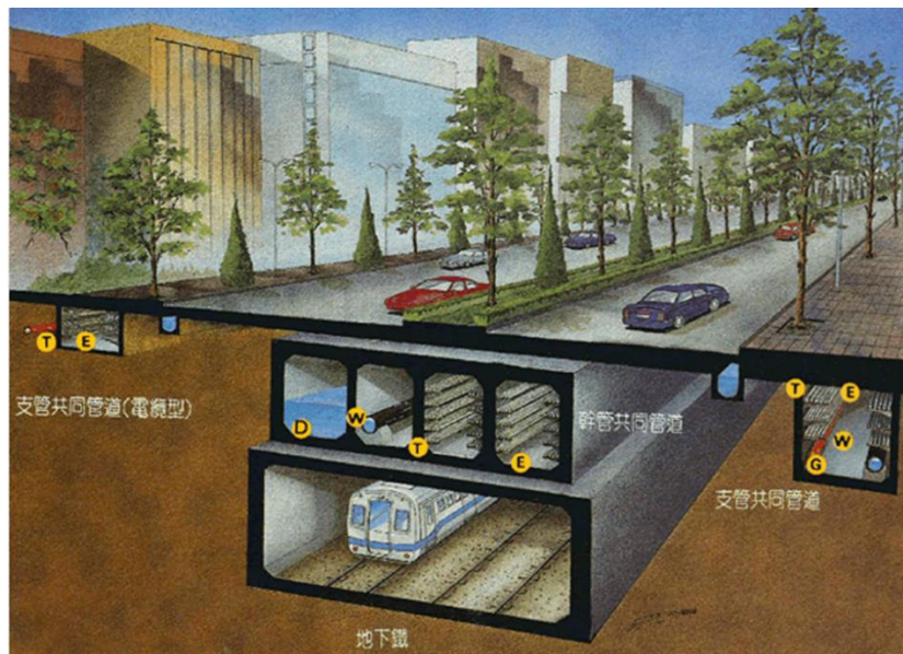
圖4.6.2.2-1 共同管線及分歧部示意圖(參考”松山線共同管道工程規劃設計理念”)
