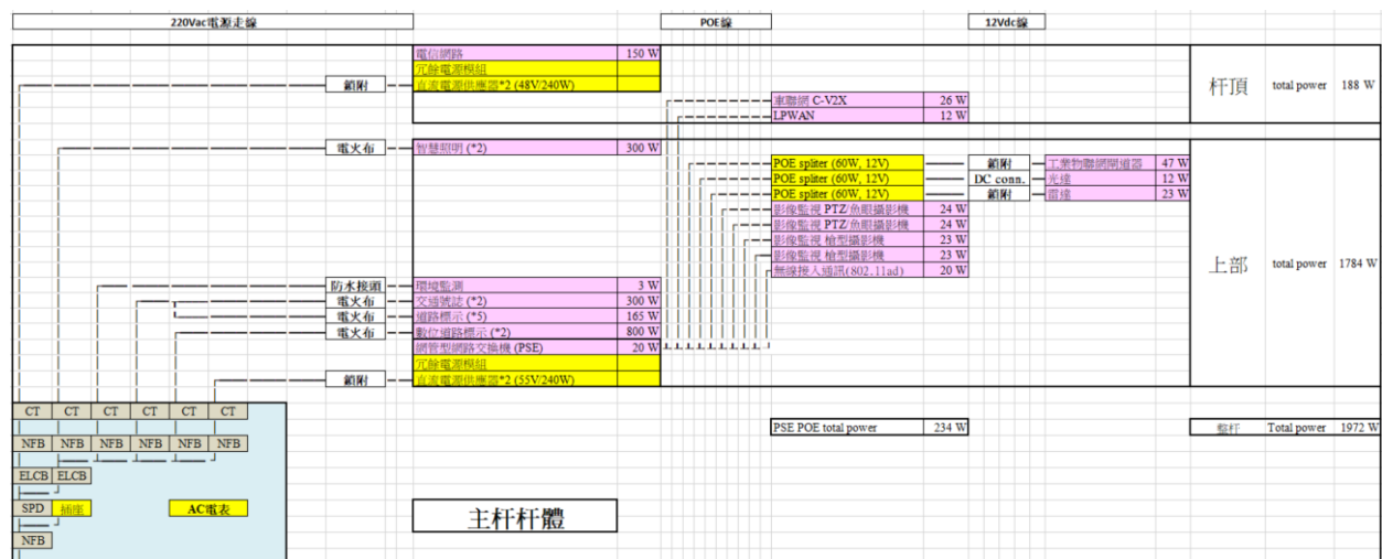
圖5.4.1-1 Type 2供電網路圖
