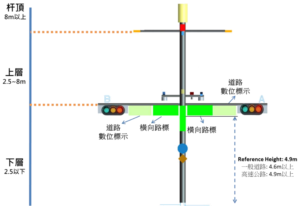
圖 4.5.1.1-4 Type 2 懸掛式掛載設備示意圖
