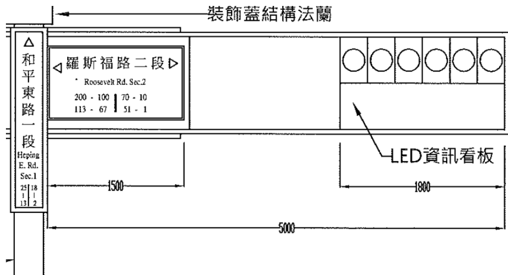
圖 4.5.1.1-5 台北市工務局交通號誌設計參考 (引用臺北市政府工務局「公園路燈工程管理處臺北市路燈、號誌桿件附掛設施共桿整合專業服務總結報告」)
