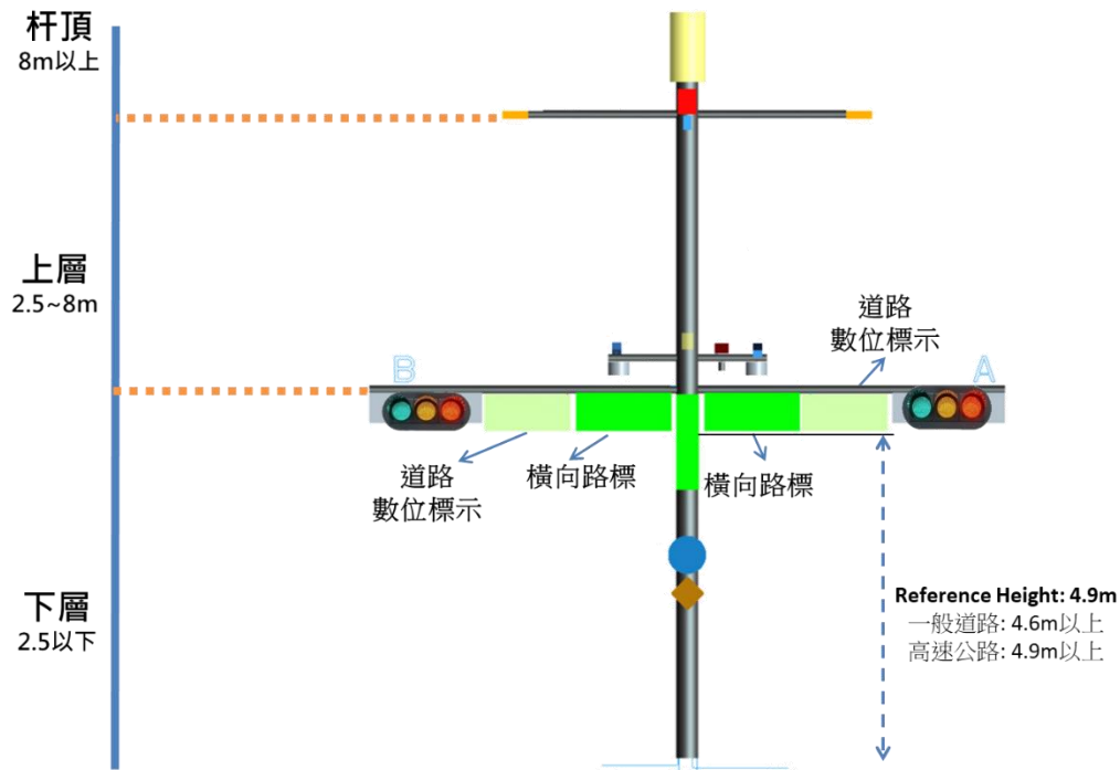
圖 4.1.4.1.1-6 Type 2 懸掛式掛載設備示意圖
