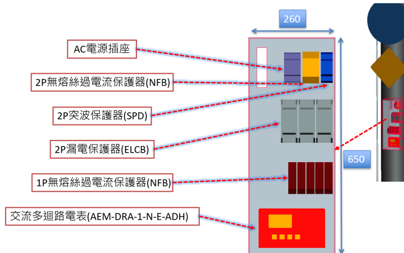
圖 5.4.3-2 Type 4 分電盤配置圖
